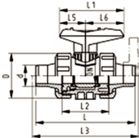
DN10/15 - 50
